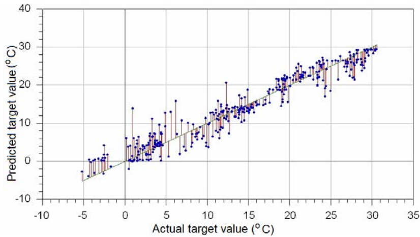
Fig. 3 – Predicted target values vs. actual target values in Model 1.
